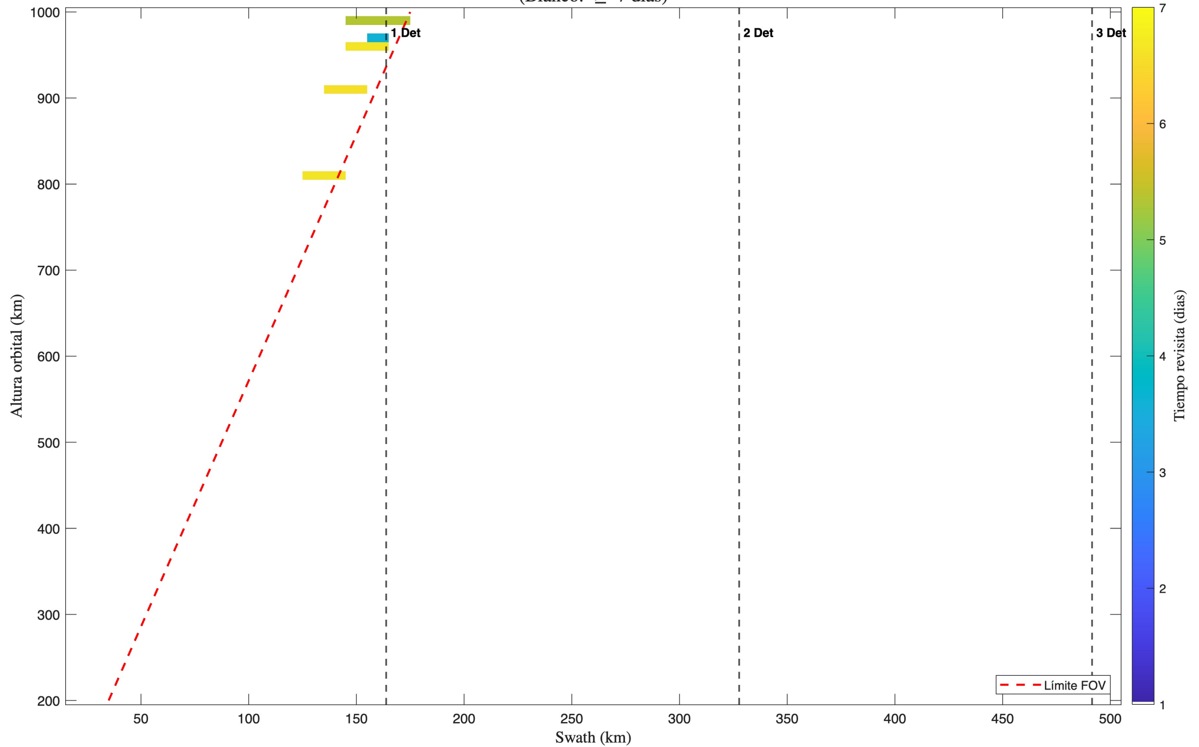
Tiempo Revisita - 3 Satellite(s); 1 Telescopio(s): Refractivo; Detector 2 (Blanco: \geq 7 días)
